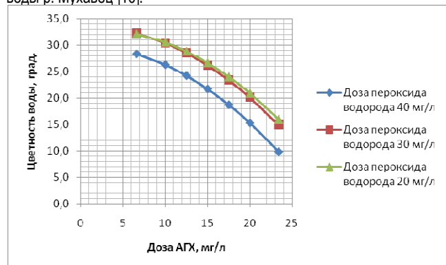
Рис. 1. Влияние дозы АГХ на остаточную цветность воды р. Мухавец при различных дозах пероксида водорода
