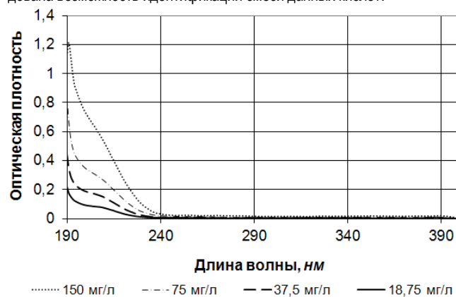
Рис. 14. Спектры поглощения водного раствора смеси муравьиной, уксусной и пропионовой кислот в равных пропорциях
