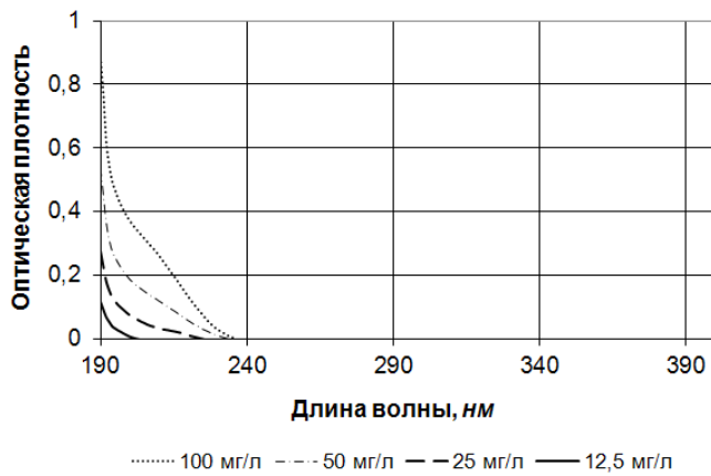
Рис. 8. Спектр поглощения водного раствора янтарной кислоты
