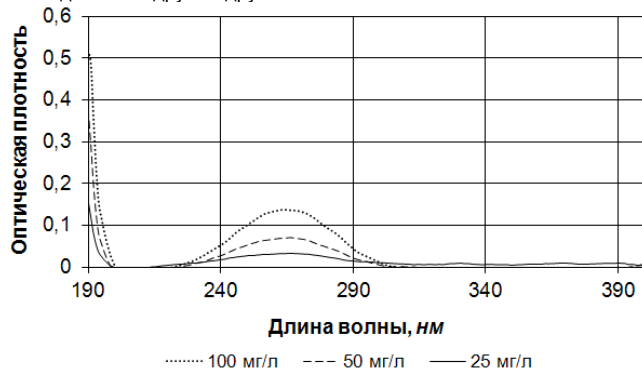
Рис. 11. Спектр поглощения водного раствора ацетона
