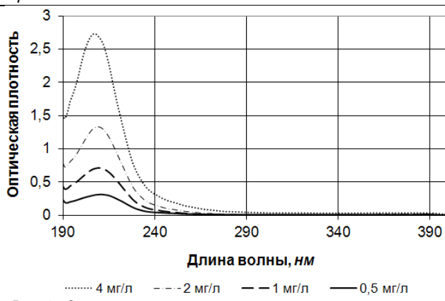
Рис. 10. Спектр поглощения водного раствора яблочной кислоты
