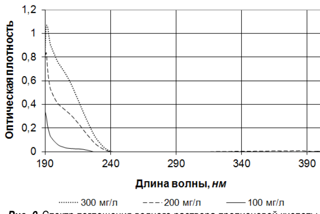
Рис. 9. Спектр поглощения водного раствора пропионовой кислоты
