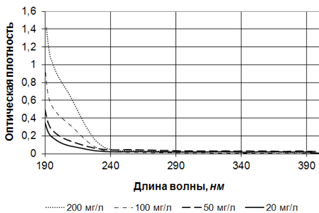
Рис. 7. Спектр поглощения водного раствора уксусной кислоты
