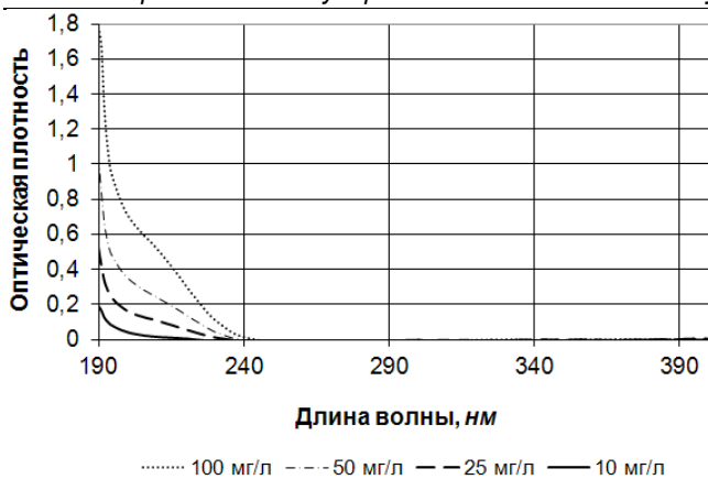
Рис. 6. Спектр поглощения водного раствора лимонной кислоты
