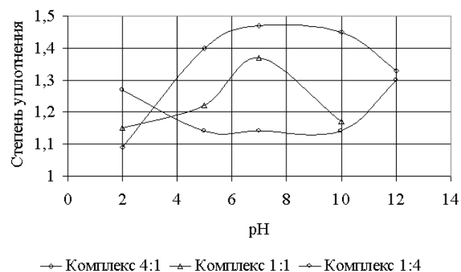
Рис. 2. Степень уплотнения агрегата в зависимости от pH раствора
